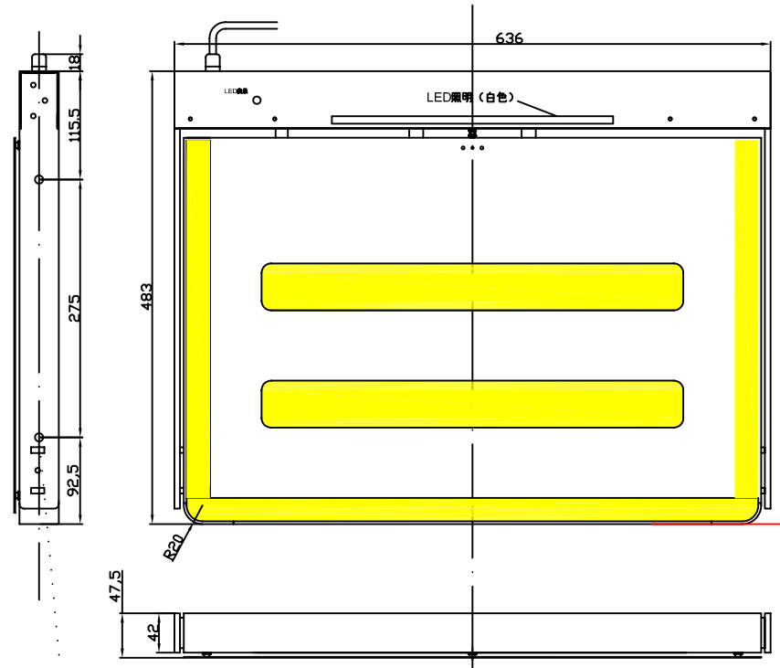
格納寸法
